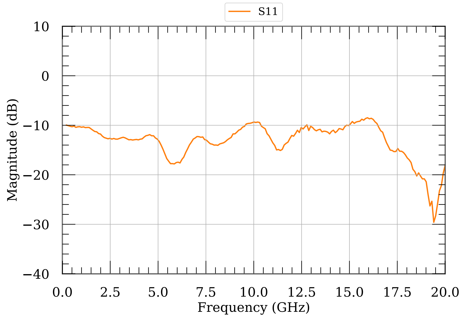
LNA S-params module031
